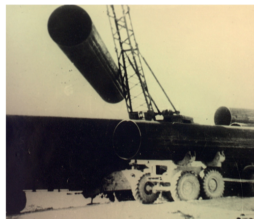
Строительство магистрального газопровода Челябинск–Петровск
